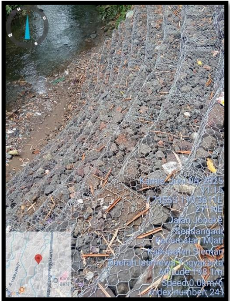
Bronjongisasi sungai
